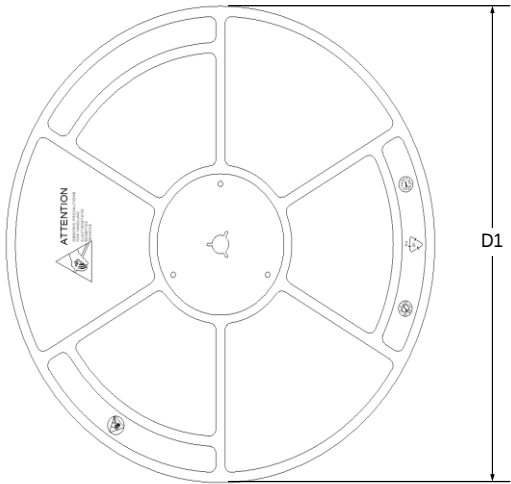
REEL DIMENSIONS
